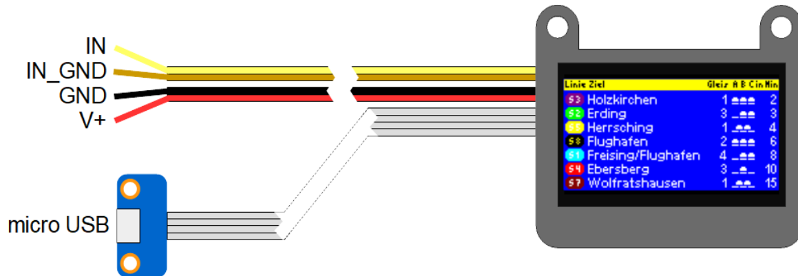
Abb. 11: Anschlussübersicht
