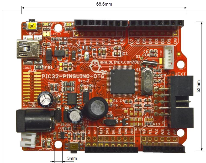
Abb. 27: Abmessungen Steuerplatine
