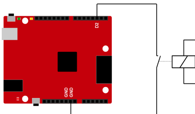
Abb. 24: Anschluss eines Relais
