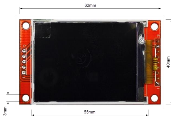
Abb. 26: Abmessungen Display
