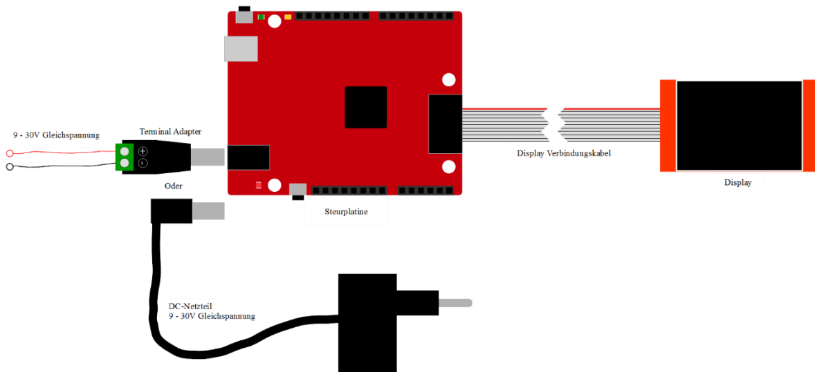
Abb. 17: Anschluss aller Komponenten im einfachsten Betriebsmodus
