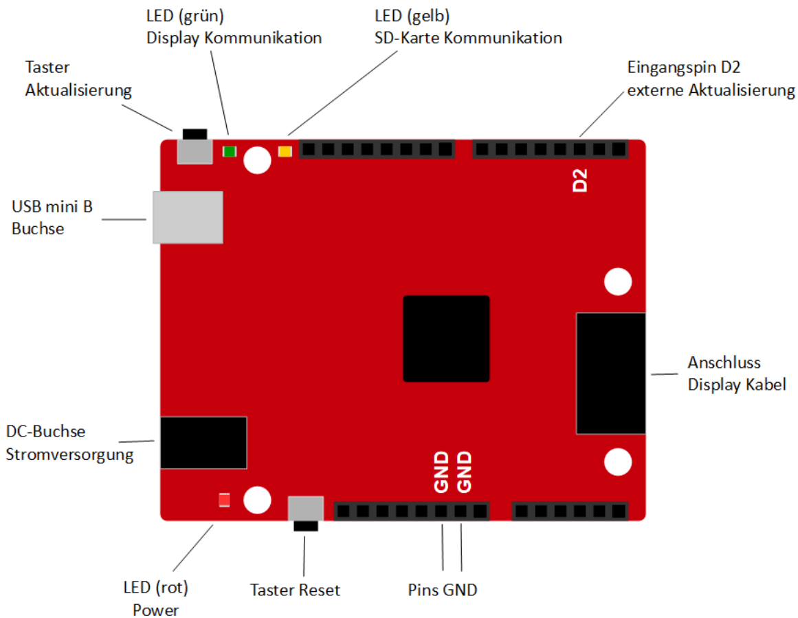
Abb. 21: Übersicht Steuerplatine
