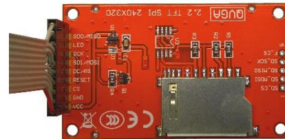
Abb. 23: Anschluss Kabel
