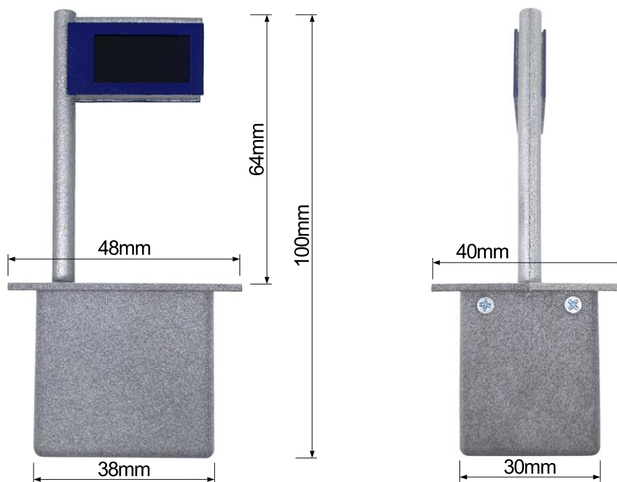
Abb. 46: Abmessungen Modell
