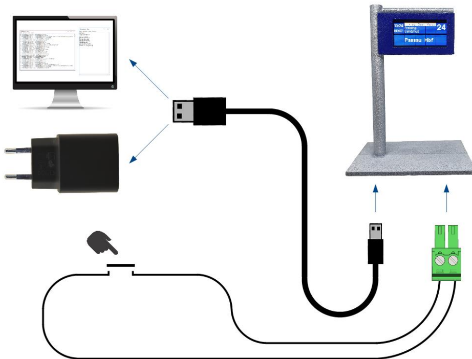
Abb. 45: Anschlussübersicht
